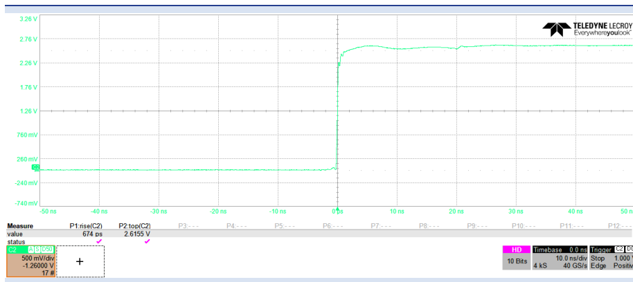
上升时间
